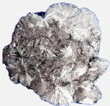
▲ 黑磷
