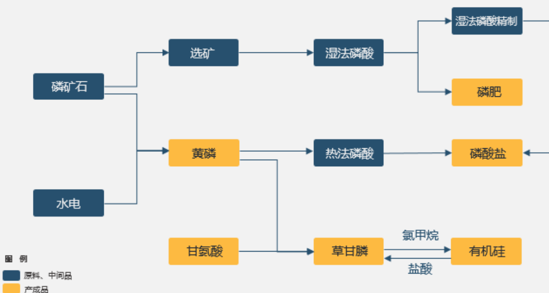
▲ 矿电化一体
