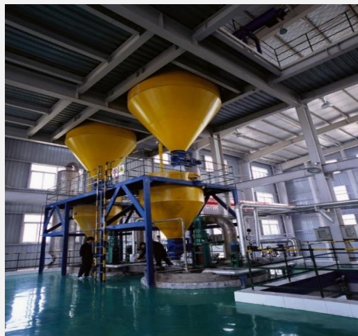
▲ 装置改造
