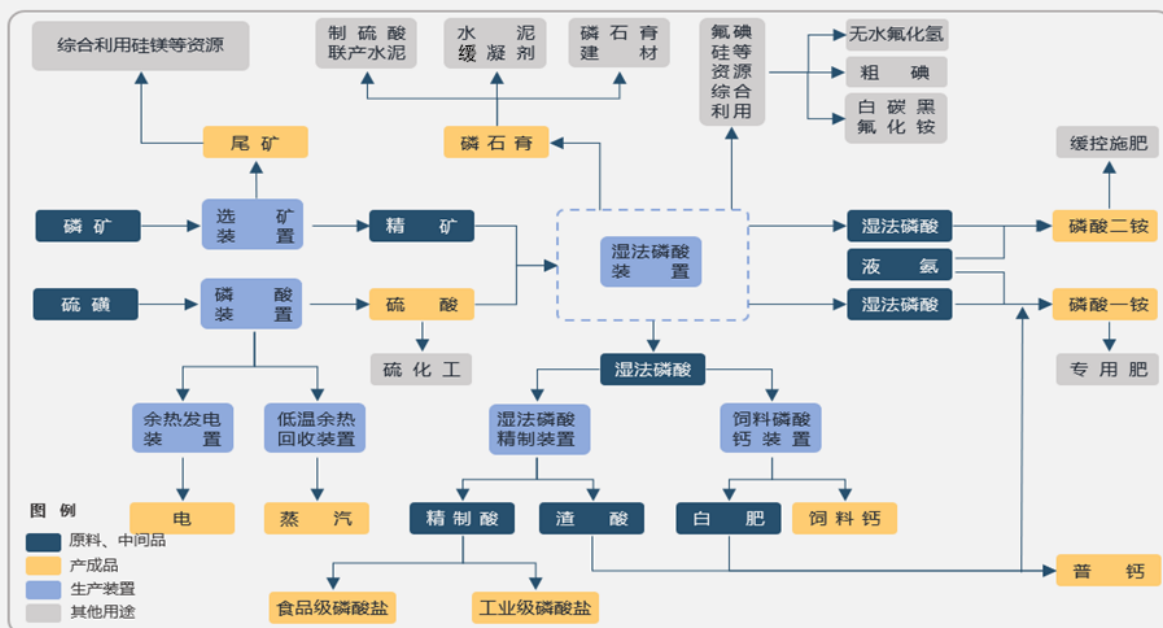
▲ 矿肥化结合
