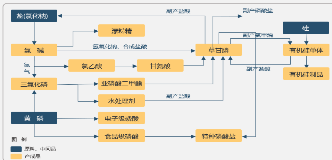
▲ 磷硅盐协同
